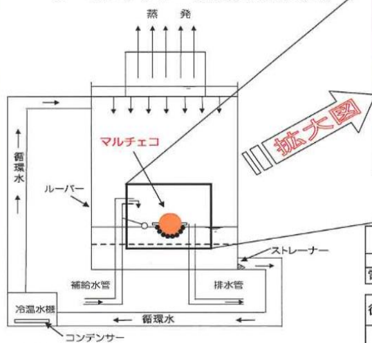
クーリングタワー概念図（断面図）
